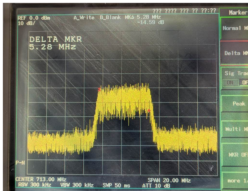
Fig3.受信スペクトラム
