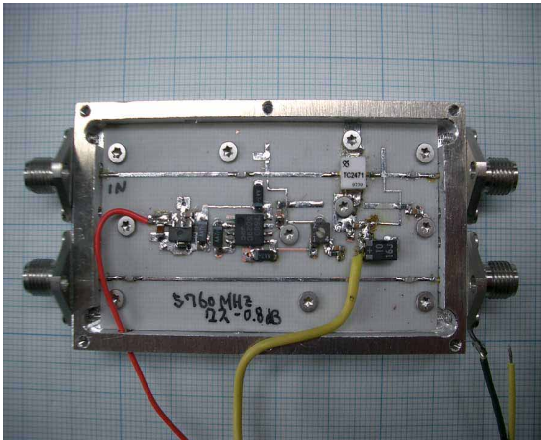
自作試作基板送信アンプ試作(500mW)
