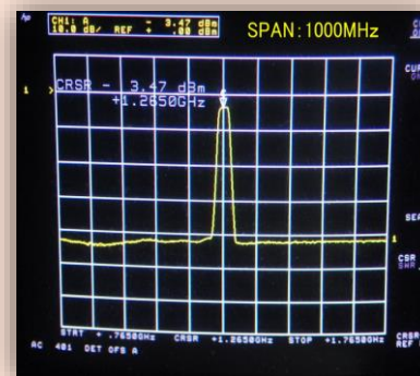
SPAN : 1000MHz
