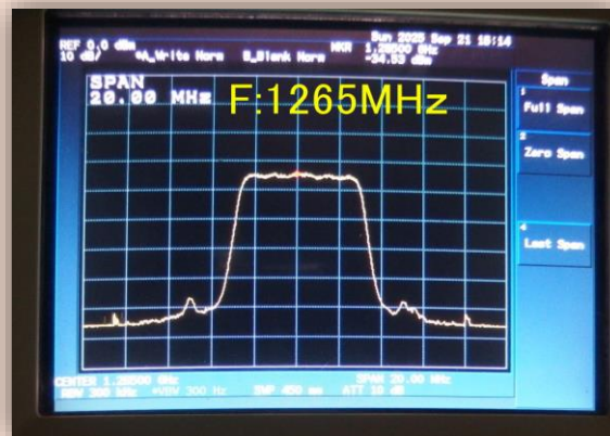
SPAN : 20MHz (1265MHz)
